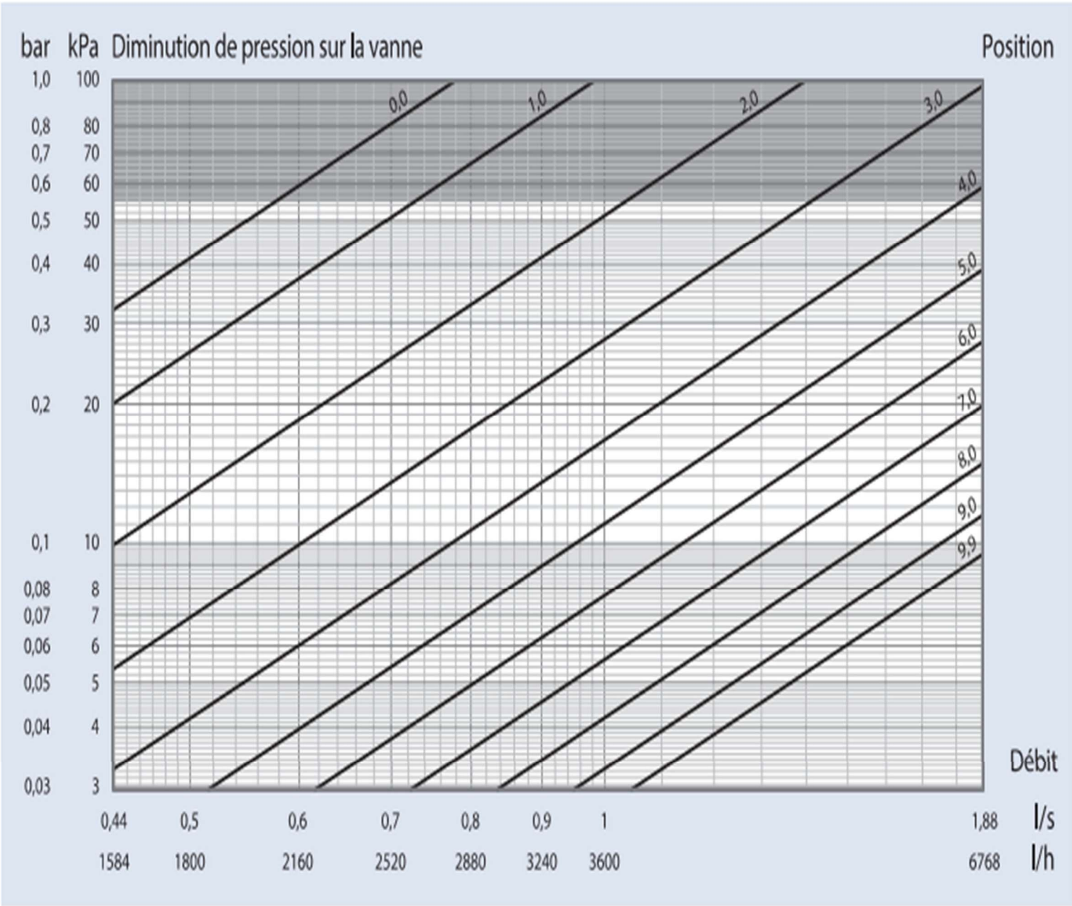
DN 40H - Débit élevé
